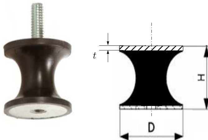
Abbildung 1: Gummi–Rundpuffer
